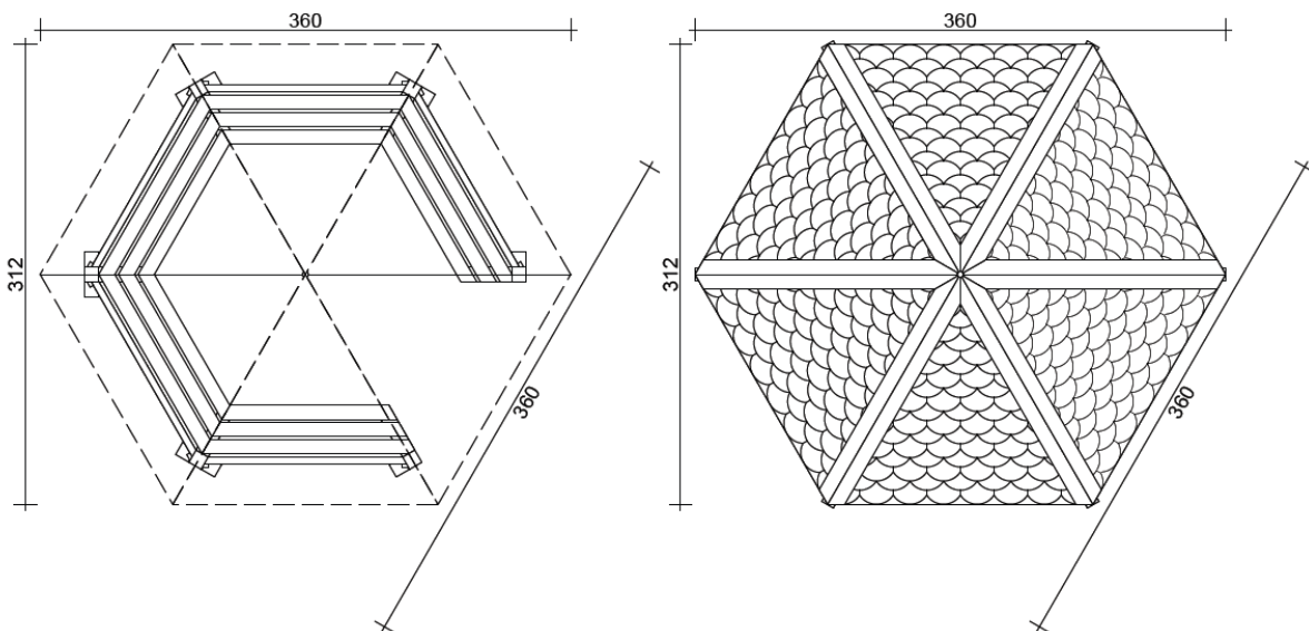
Κάτοψη Παγκάκι, Κάτοψη Κiosκι (Διαστάσεις σε cm).
